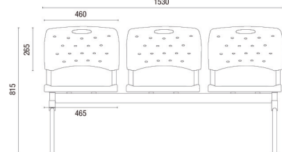
35.010 VIVA BANQUETA ANCHO SIN BRAZOS 2 PUESTOS - 1025 MM 3 PUESTOS - 1530 MM 4 PUESTOS - 2050 MM 5 PUESTOS - 2575 MM
