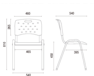
35.008 P VIVA MULTIUSO
