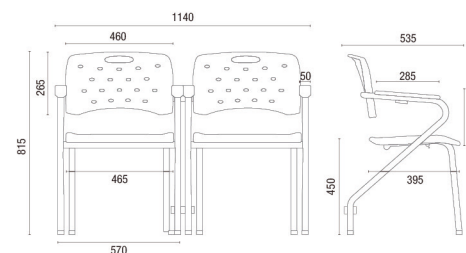
35.007 Z VIVA MULTIUSO MECANISMO DE UNIÓN
