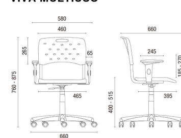
35.004 VIVA GIRATORIA CON BASE DE ACERO
