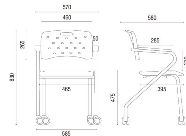
35.007 Z ROD VIVA MULTIUSO CON RUEDAS
