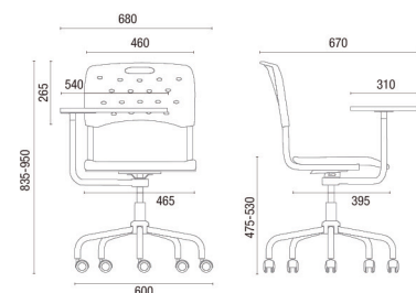
35.004 VIVA GIRATORIA TABLERO 360°
