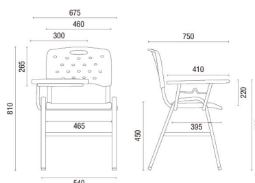
35.008 PU VIVA UNIVERSITARIA
