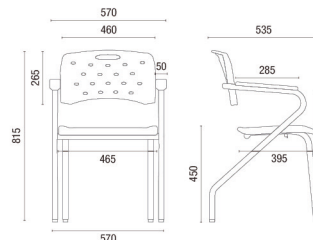
35.007 Z VIVA MULTIUSO
