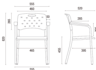
35.007 P VIVA MULTIUSO
