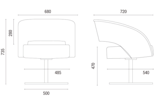
36010 SPOT SILLÓN DE ESPERA BASE DISCO
