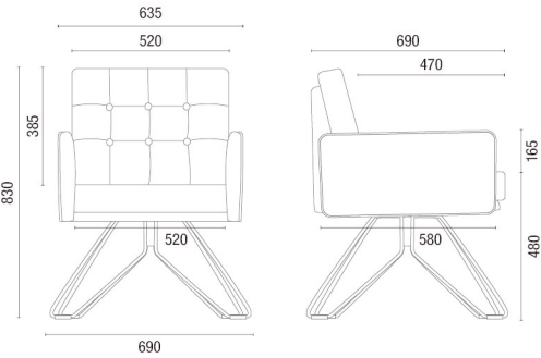
36050 SPOT SILLÓN DE ESPERA
