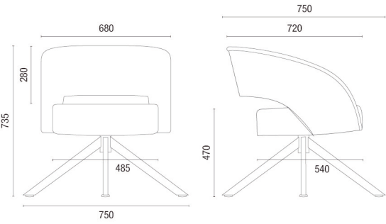
36010 SPOT SILLÓN DE ESPERA 4 PATAS
