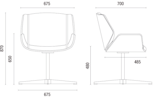
36060 SPOT SILLÓN DE ESPERA
