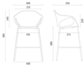
33120 STAY TABURETE
