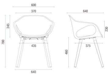
33206 STAY MULTIUSO
