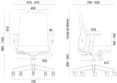
40.101 IDEA EJECUTIVA ALTA SYCRON RP BRAZOS ID BASE ALUMINIO
