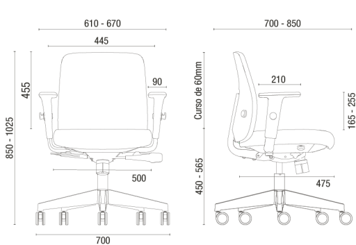
40.102 / 40.202 IDEA GIRATORIA MEDIANA SYCRON RP BRAZOS ID BASE ALUMINIO
