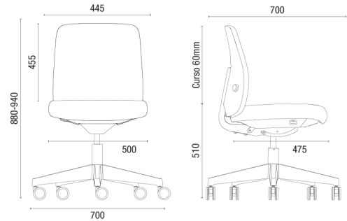
40.202 SR IDEA GIRATORIA MEDIANA PLATAFORMA GIRATORIA BASE NYLON
