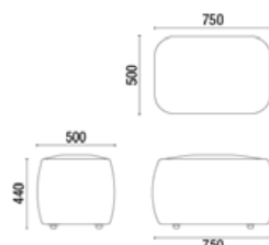
26.211 BLOKZ ASIENTO 1 C 750MM
