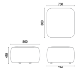
26.221 BLOKZ ASIENTO 1C 750 MM
