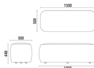
26.212 BLOKZ ASIENTO 2C 1300MM
