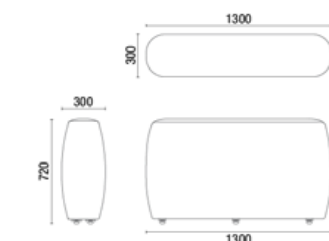
26.232 BLOKZ RESPALDO 2C 1300 MM
