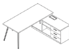
EDGE EJECUTIVO CON CAGINETE LATERAL LARGO: 1800 - 2200 MM ALTURA TOTAL: 750 MM PROFUNDIDAD: 700 - 1000 MM
