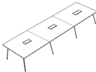
EDGE MESA REUNIÓN RECTA 12 - 14 PUESTOS LARGO: 3800 - 4600 MM ALTURA TOTAL: 750 MM PROFUNDIDAD: 1400 MM
