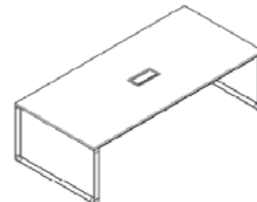
QUALITY MESA DE REUNIONES 4 - 6 PUESTOS LARGO: 1400 - 2400 MM ALTURA TOTAL: 750 MM PROFUNDIDAD: 800 - 1200 MM
