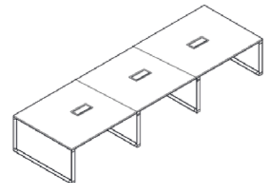
QUALITY MESA DE REUNIONES 8 - 10 PUESTOS LARGO: 2600 - 3600 MM ALTURA TOTAL: 750 MM PROFUNDIDAD: 1200 - 1400 MM
