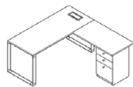
QUALITY EJECUTIVA CON CAJONERA LAETRAL LARGO: 1400 - 2000 MM ALTURA TOTAL: 750 MM PROFUNDIDAD: 700 - 1000 MM
