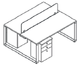
QUALITY BENCH 2 PUESTOS LARGO: 1200 - 1800 MM ALTURA TOTAL: 750 MM PROFUNDIDAD: 1200 - 1400 MM
