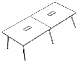
SILHOUETTE MESA REUNIÓN RECTA 8 - 10 PUESTOS LARGO: 2600 - 3600 MM ALTURA TOTAL: 750 MM PROFUNDIDAD: 1200- 1400 MM
