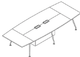
SILHOUETTE MESA REUNIÓN CURVA 10 PUESTOS LARGO: 3.600 MM ALTURA TOTAL: 750 MM PROFUNDIDAD: 1.400 MM
