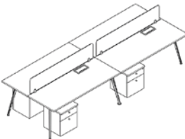
SILHOUETTE BENCH 4 PUESTOS LARGO: 2400 - 3600 MM ALTURA TOTAL: 750 MM PROFUNDIDAD: 1200 - 1400 MM
