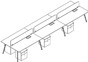
SILHOUETTE BENCH 6 PUESTOS LARGO: 3600 - 5400 MM ALTURA TOTAL: 750 MM PROFUNDIDAD: 1200 - 1400 MM
