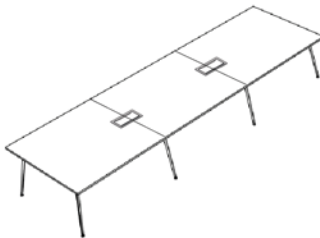
SILHOUETTE MESA REUNIÓN RECTA 12 - 14 PUESTOS LARGO: 3800 - 4600 MM ALTURA TOTAL: 750 MM PROFUNDIDAD: 1400 MM
